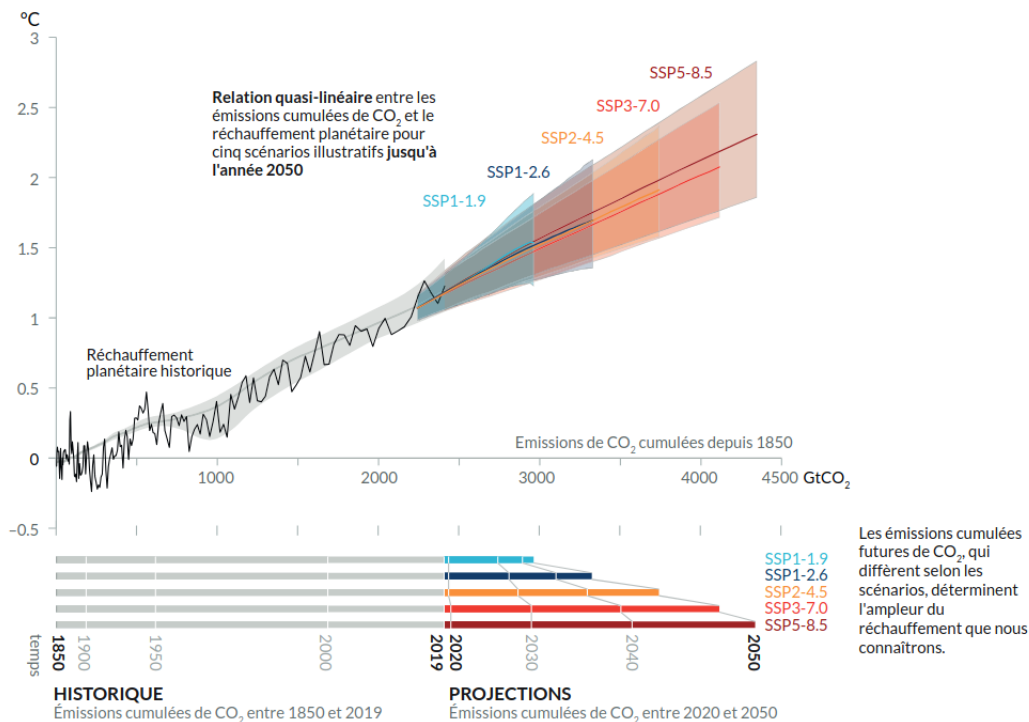
Augmentation de la température à la surface du globe depuis 1850-1900 (°C) en fonction des émissions cumulées de CO 2 (GtCO 2 )
